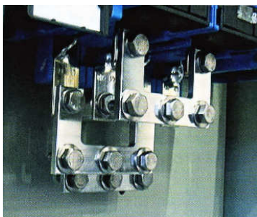
شکل ۱۷،۲- اتصالات کابل
