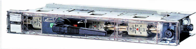
شکل ۱۴،۸ - فیوز کلید NH مدل رک
