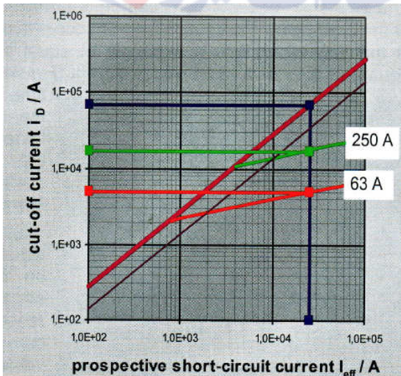
شکل ۲،۶ - منحنی قطع
