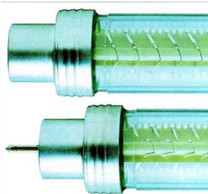
شکل ۴،۵- فیوزهای Full Range
