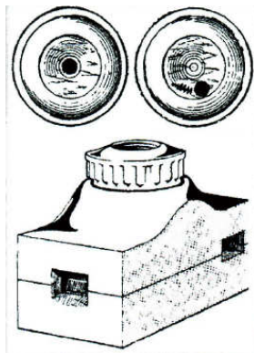
شکل ۱، ۲، فیوزهای نوع Diazed ساخته شده توسط برادران زمینس در سال ۱۹۰۶
