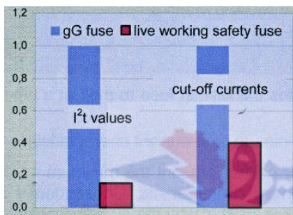
شکل ۱۶,۲ - مقادیر قطع جریانی
