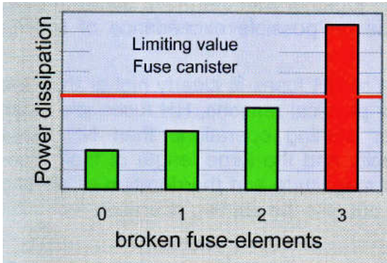
شکل ۱۱.۴- اثرات دمایی المنتهای فیوزی ذوب شده
