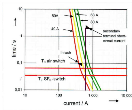
شکل ۱۱،۳- انتخاب فیوز مطابق با VDE 0671,Part 105
